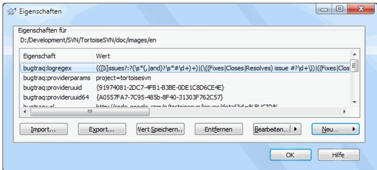
Abbildung 4.35. Subversion Eigenschaftsseite
