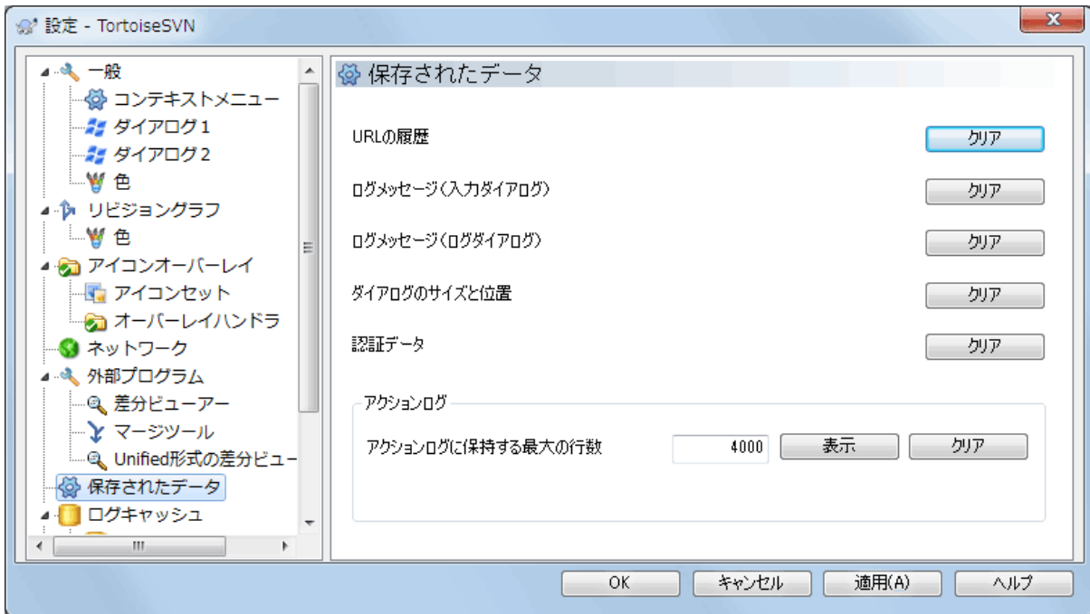
図4. 83 設定ダイアログの「保存されたデータ」ページ
