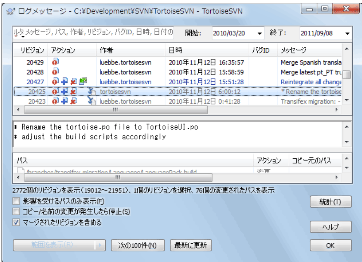
図4.22 マージ追跡リビジョンを表示したログダイアログ
