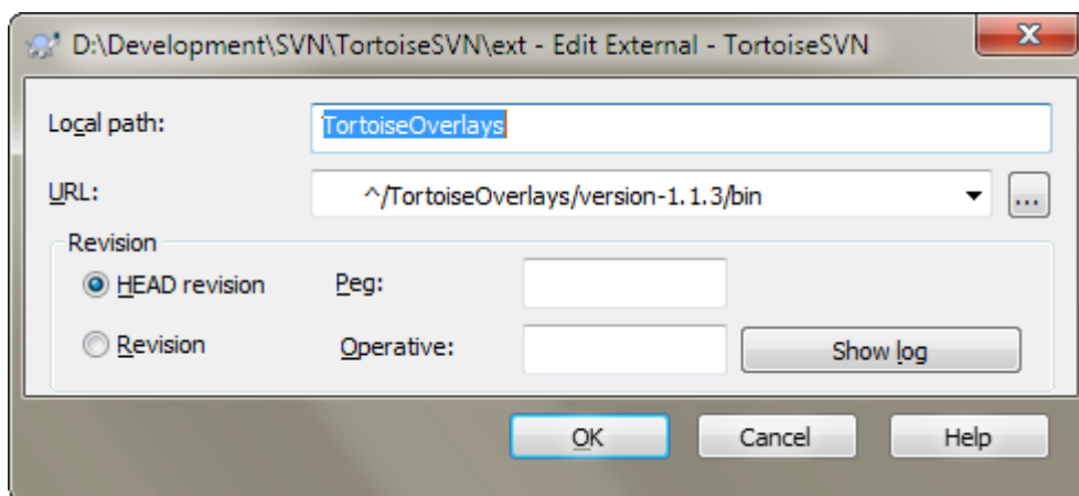
Slika 4.41. svn:externals property page
