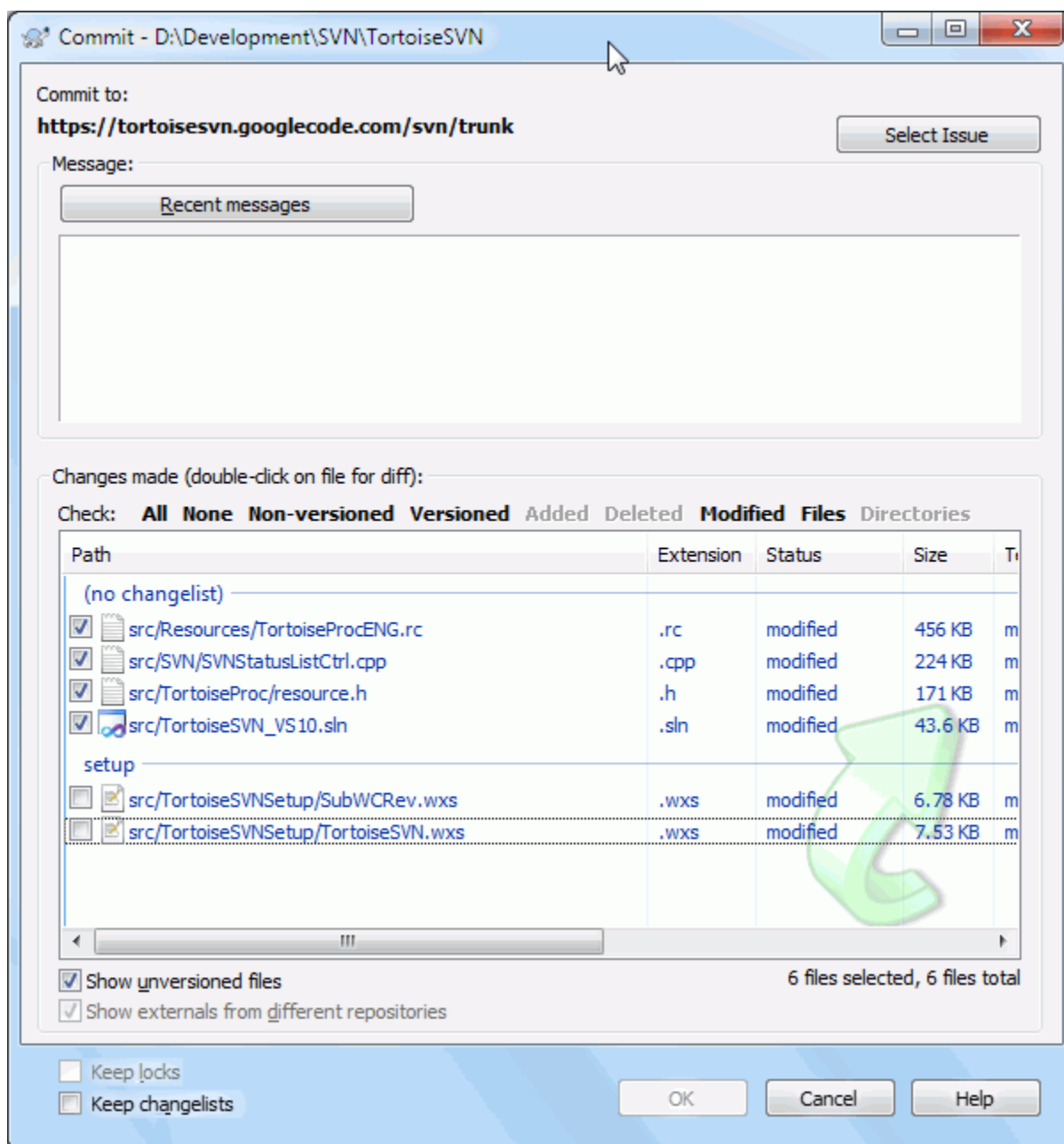
Slika 4.15. Okno za objave s sezname sprememb
