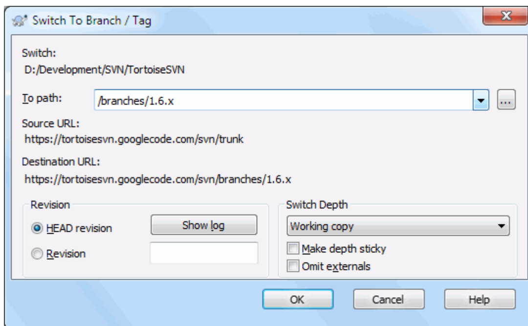
Slika 4.52. Okno za preklop
