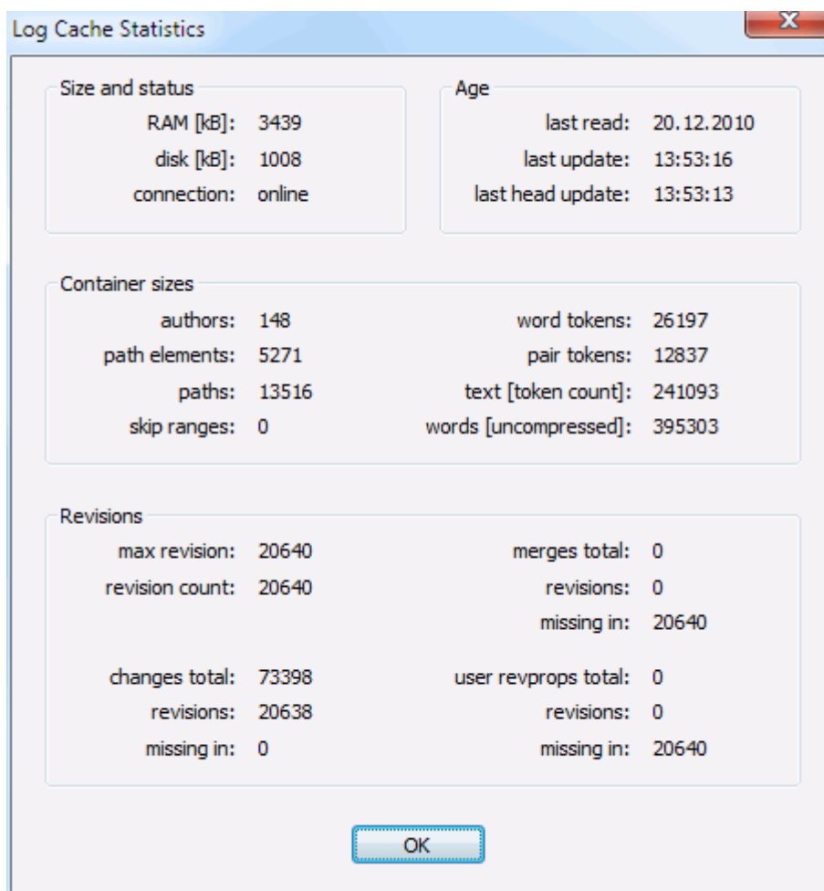
Slika 4.84. Okno nastavitve, Statistika predpomnilnika dnevnika
