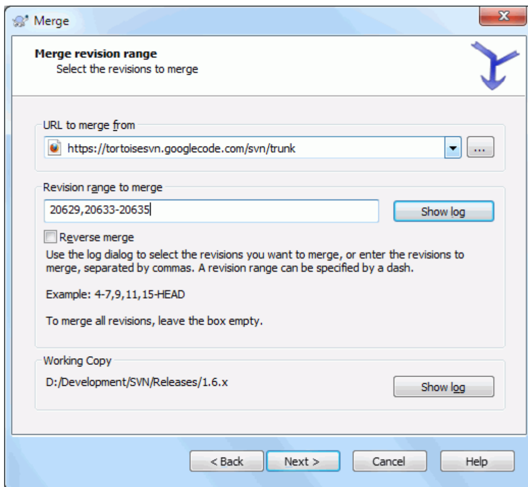
Slika 4.53. Čarovnik za spajanje - Izberite obseg revizije
