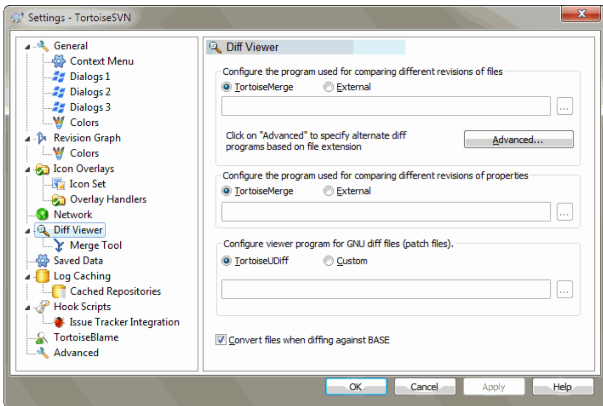
Slika 4.80. Okno nastavitve, ogledovalnik razlik
