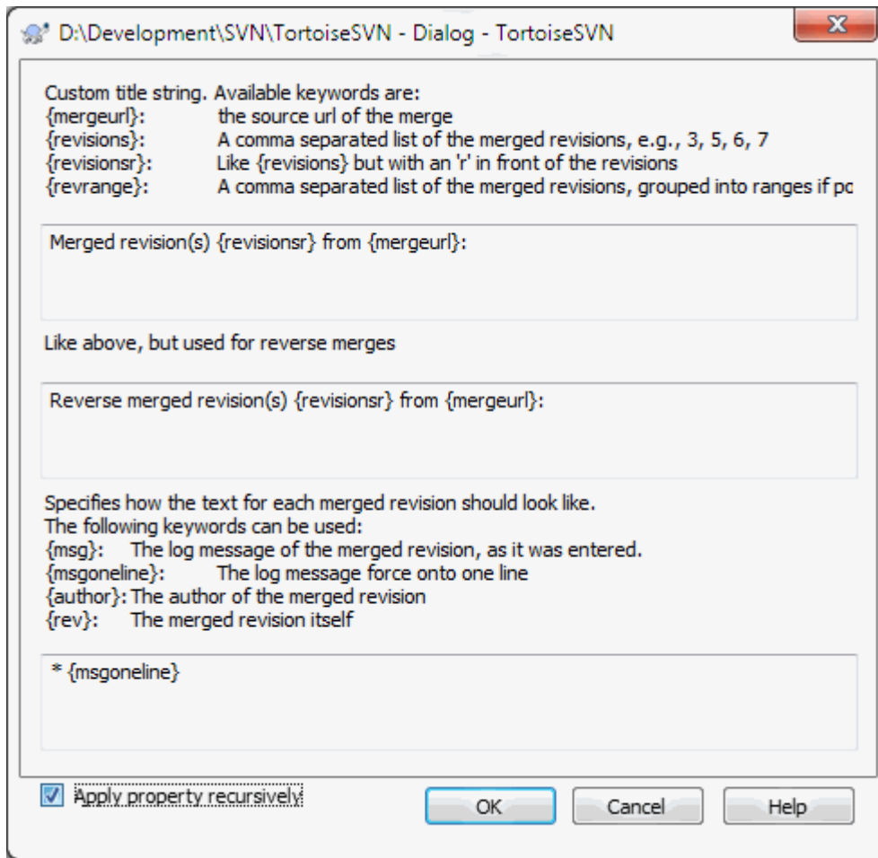
Slika 4.50. Property dialog merge log message templates
