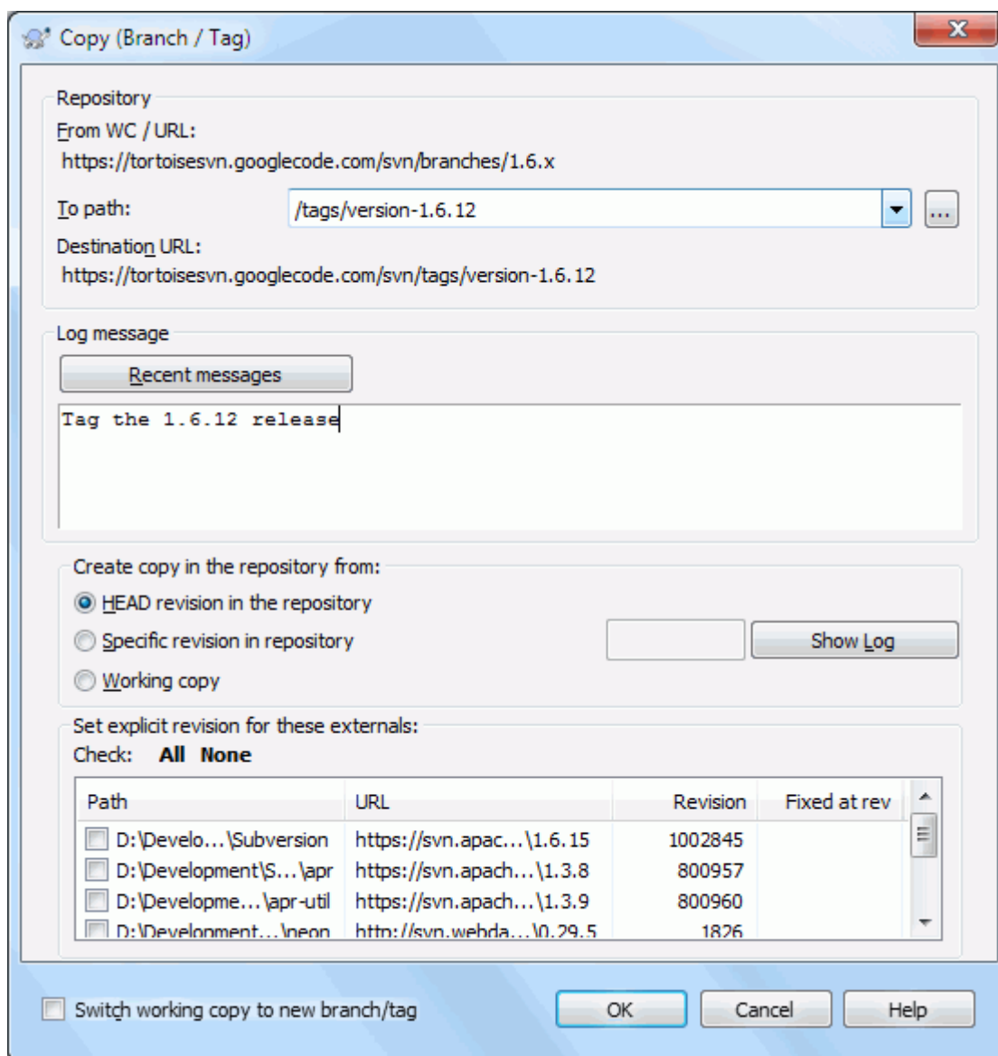
Slika 4.51. Okno za za ustvarjanje veje/oznake
