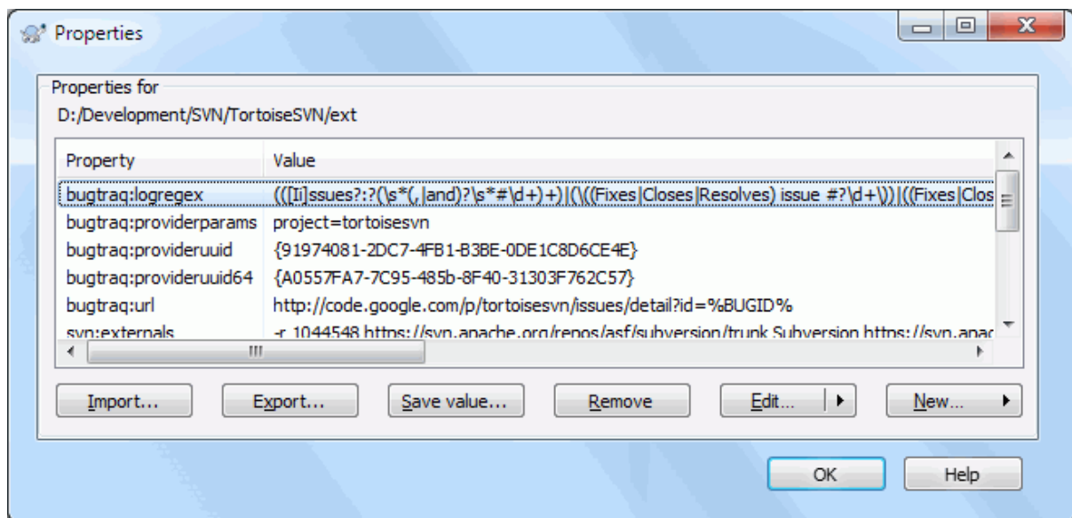
Slika 4.34. Lastnosti v sistemu Subversion
