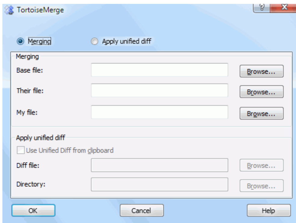
Slika 3.5. Dijalog otvaranja
