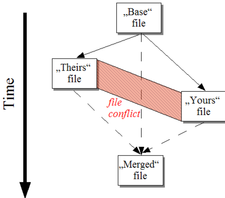
Slika 2.1. Fajl konflikt
