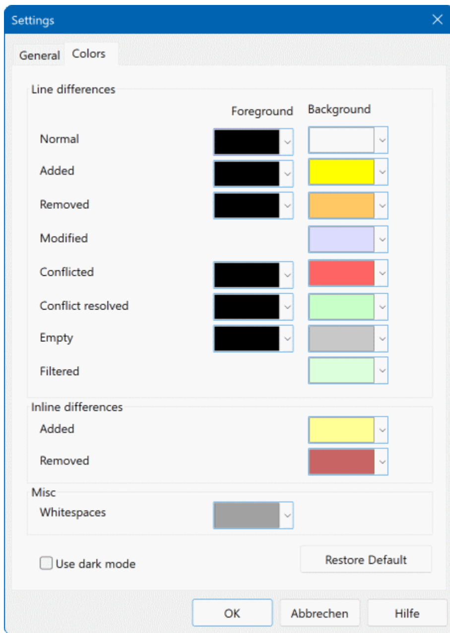
Slika 3.7. Nastavitev barv
