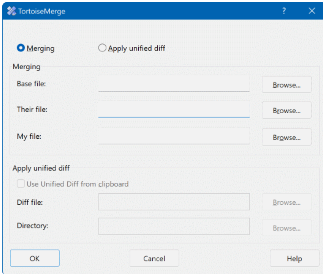
Abbildung 3.5. Der Öffnen-Dialog
