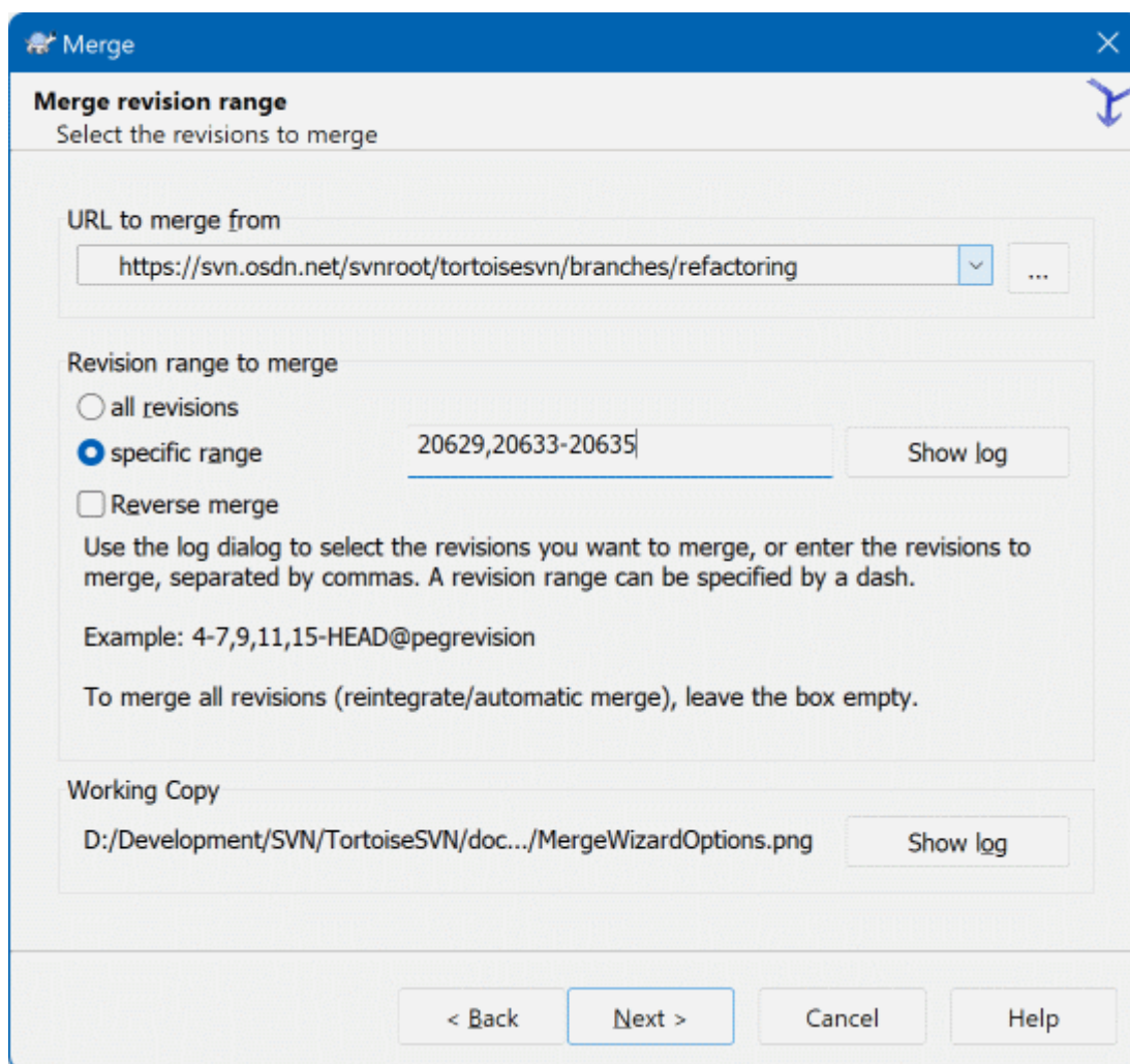
Слика 4.55. Чаробњак сојања - Избор опсега ревизија
